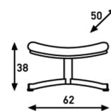
P 512: footstool non swiveling
